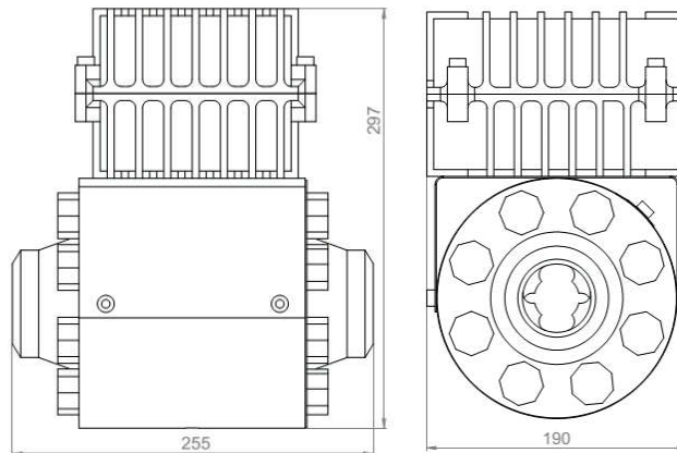
Рисунок 2.1а - Габаритные размеры бокса с УИР
