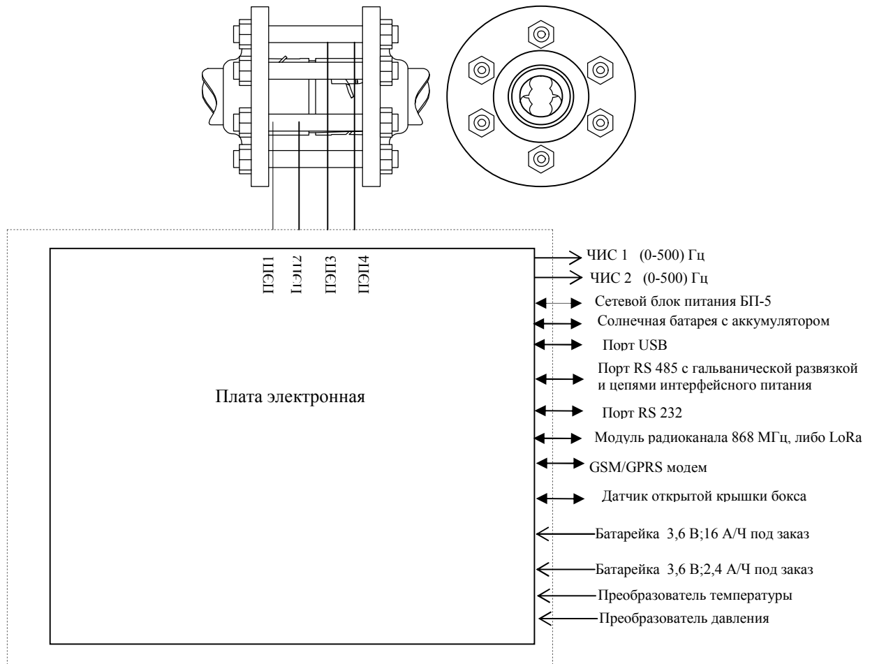
Рисунок 4.3 - Структурная схема расходомеров с УПР типа ПП 13
