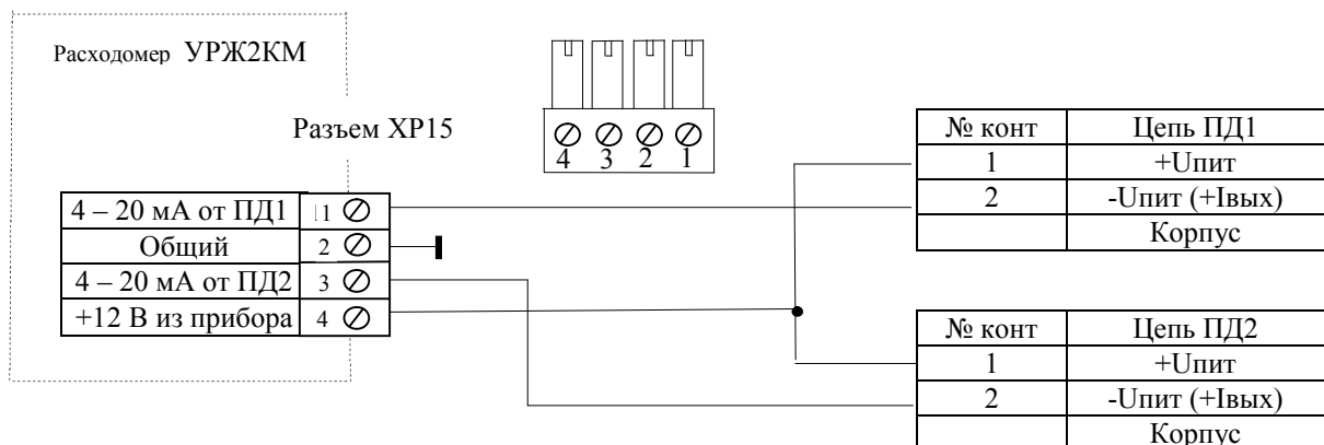
Рисунок 4.3 - Схема подключения преобразователей давления (ПД) к расходомерам
